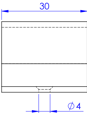
End Cap UA49349
