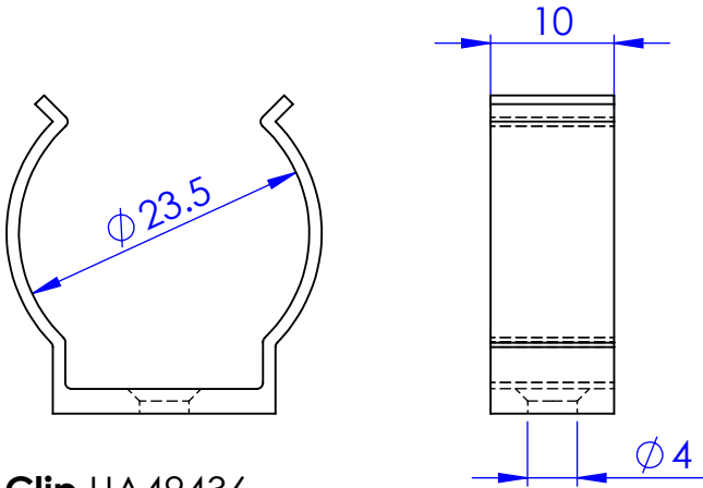
Clip UA49436
