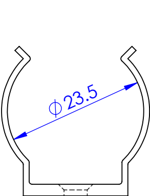
Clip UA49436
