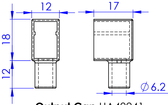
Output Cap UA49241
