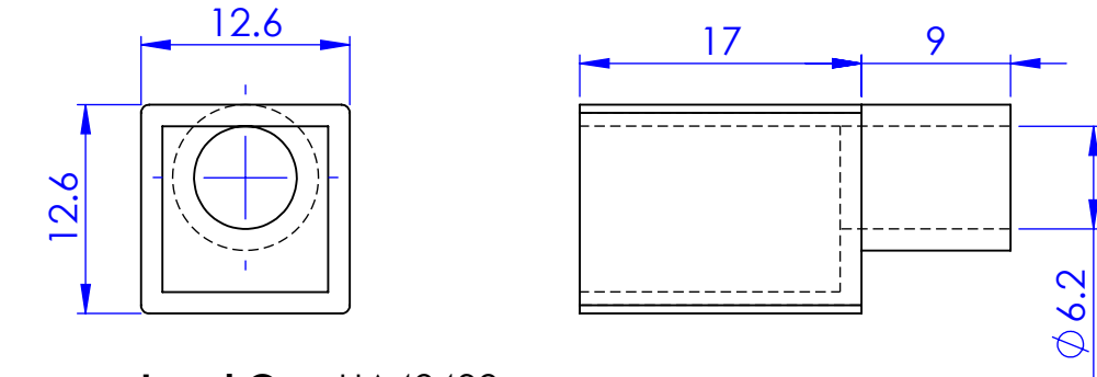
Input Cap UA49439
