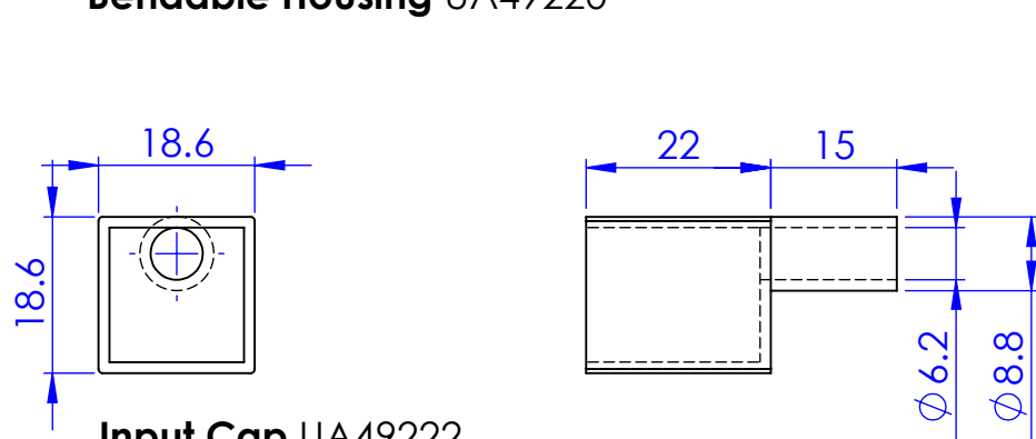
Input Cap UA49222
