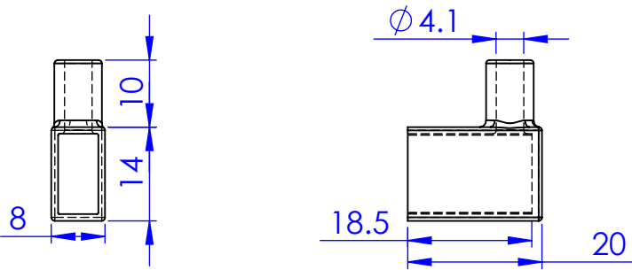
Side Cap UA49229
