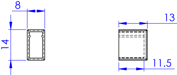
End Cap UA49227
