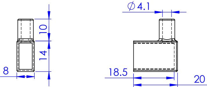
Side Cap UA49229
